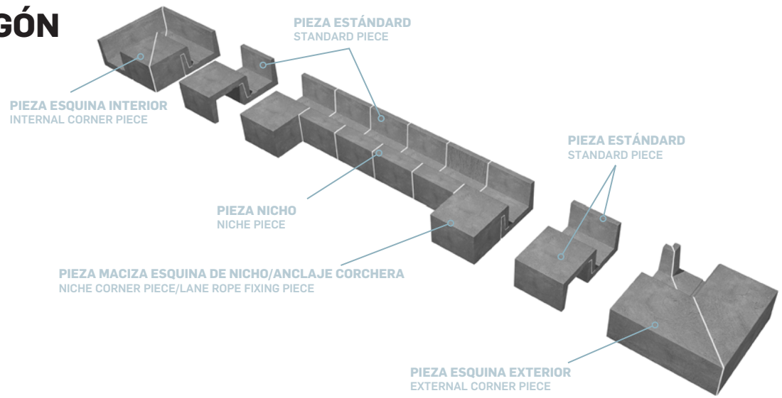
PIEZA MACIZA ESQUINA DE NICHO/ANCLAJE CORCHERA ..... NICHE CORNER PIECE/LANE ROPE FIXING PIECE Cod. 901751 [PZ255]
