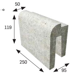
PIEZA ROMA PARA MOSAICO ..... BLUNT PIECE FOR MOSAIC Cod. 901753 [PZ135]
