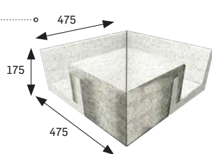
PIEZA ESQUINA EXTERIOR ..... EXTERNAL CORNER PIECE Cod. 901749 [JG745]
