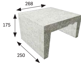
PIEZA MACIZA ESQUINA DE NICHO/ANCLAJE CORCHERA ..... NICHE CORNER PIECE/LANE ROPE FIXING PIECE Cod. 901751 [PZ255]
